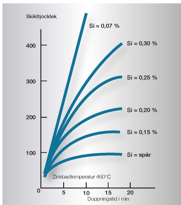
Figur 1. Förhållandet mellan dopptid och skiktthjocklek för stål med olika kiselhalter. Kurvorna är medelkurvor baserade på både studier och praktisk erfarenhet. Betydande variationer kan förekomma mellan stål med samma kiselinnehåll men från olika charger. Kurvorna gäller för ett zinkbad utan tillsats av nickel.
